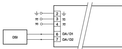
DSI PCA T5 EXCEL one4all
