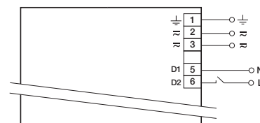
corridorFUNCTION PCA TC ECO xtrec II
