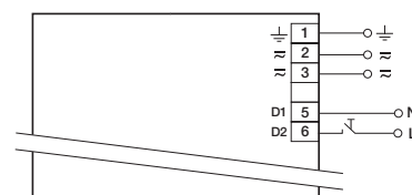
switchDIM PCA TC ECO xtrec II
