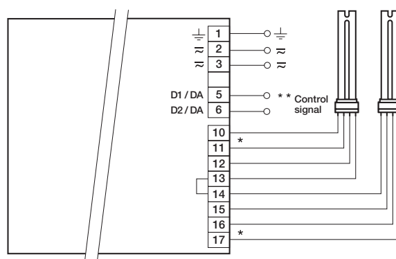
PCA TC ECO x|tec II 2x18–42 W
