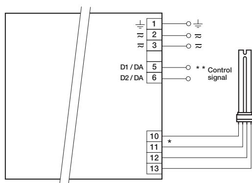
PCA TC ECO x|tec II 1x18–57 W
